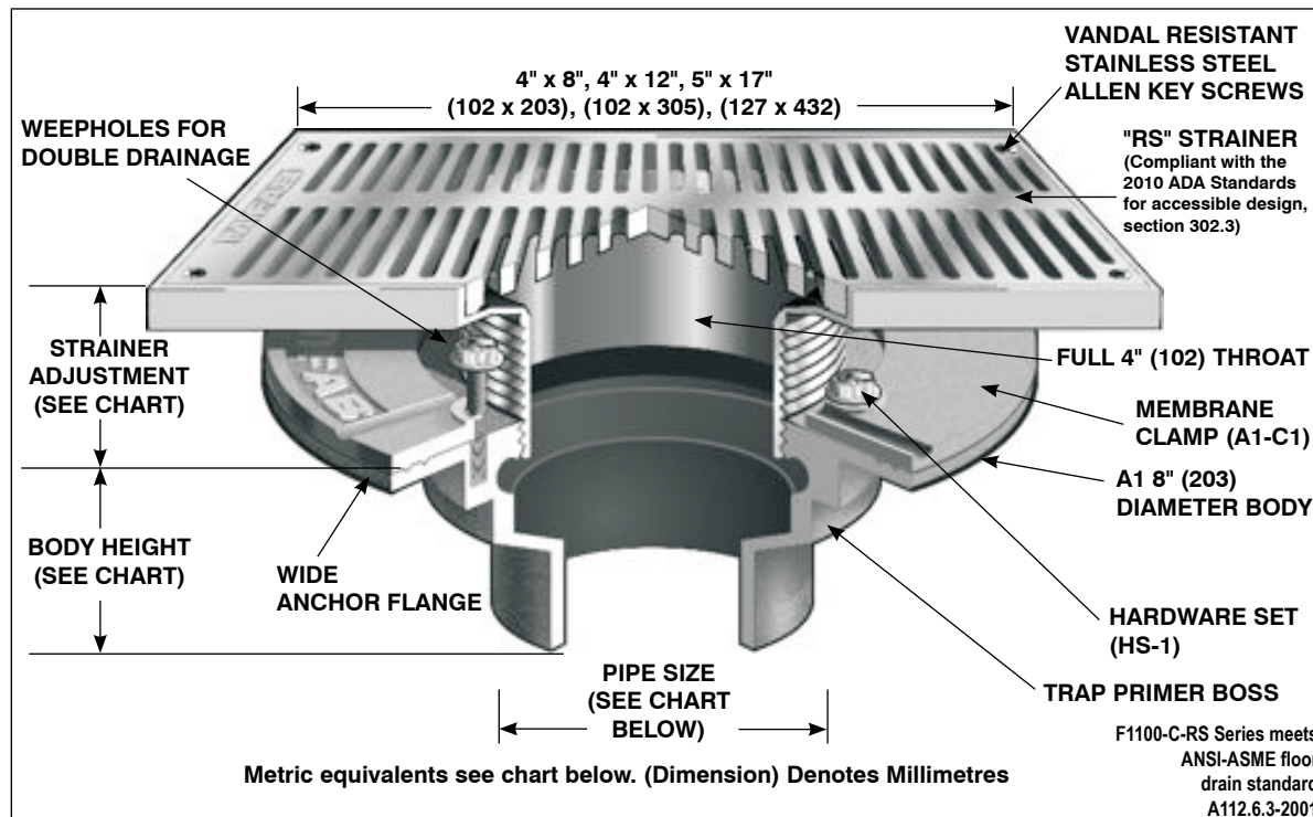
A1 BODY
