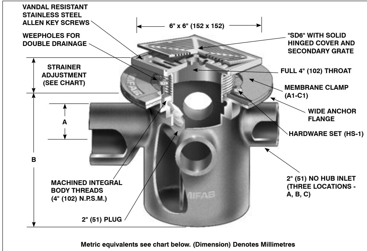
F117(*) (*) Denotes Outlet Size
