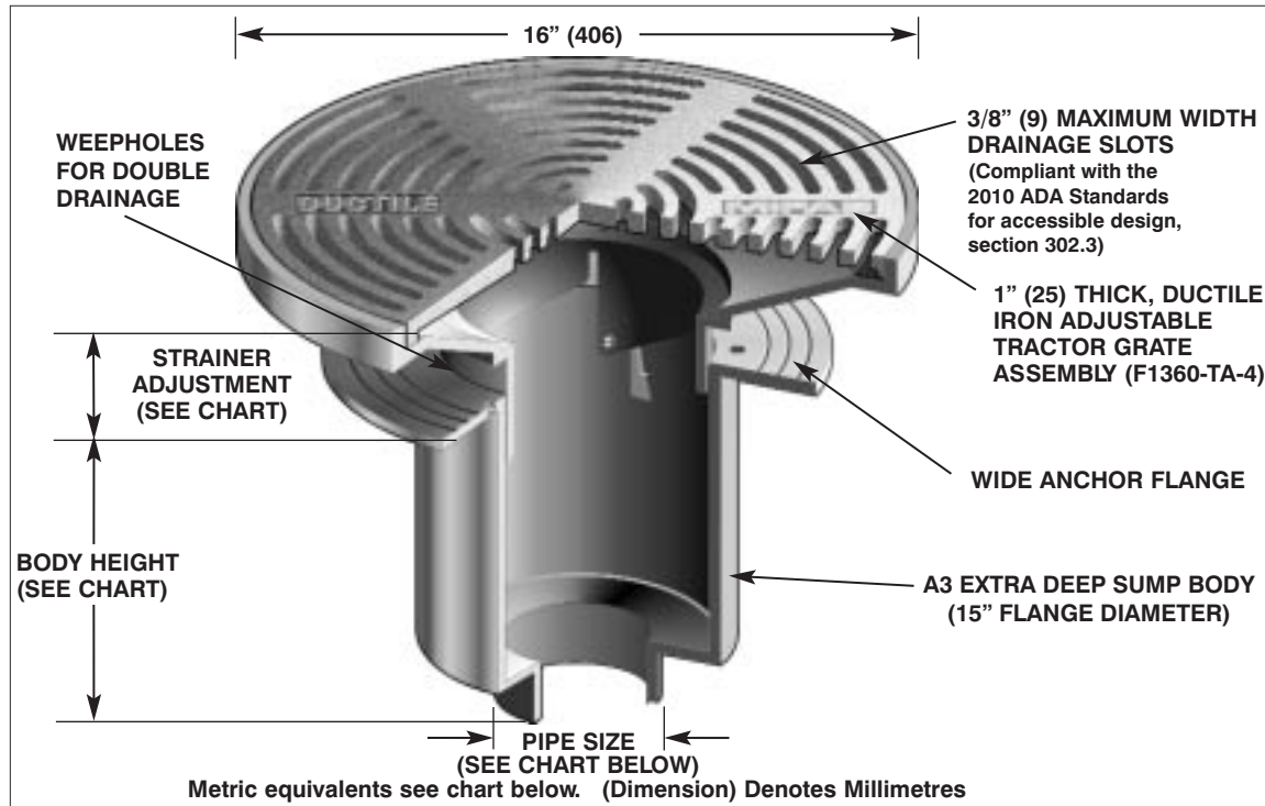
A3 Body
