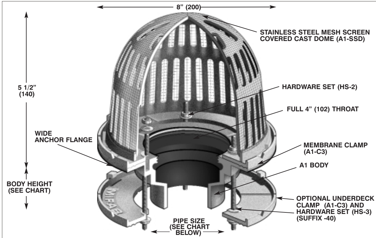
A1 BODY
